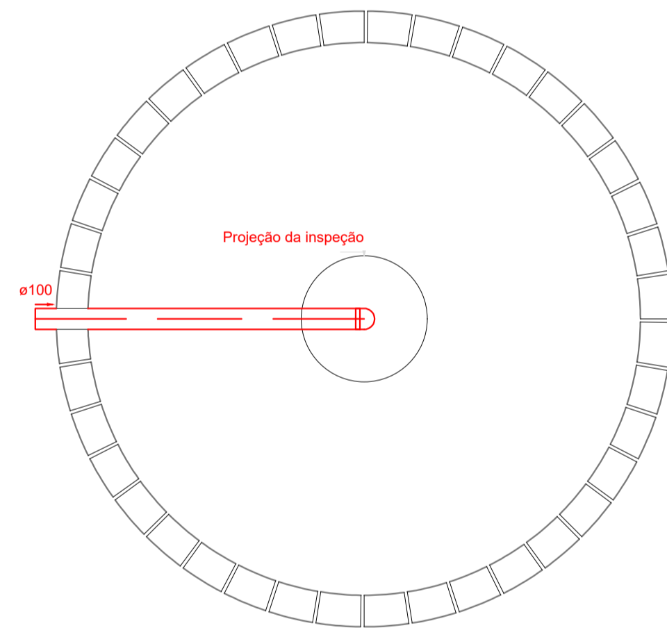
PLANTA BAIXA - SUMIDOURO ESCALA: 1/25
