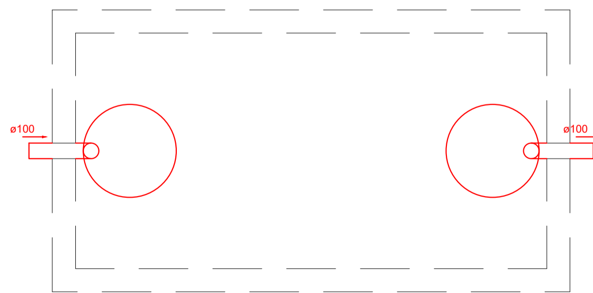
PLANTA BAIXA - TANQUE SÉPTICO ESCALA: 1/25
