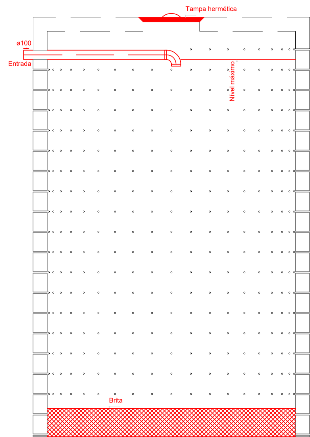
CORTE - SUMIDOURO ESCALA: 1/25
