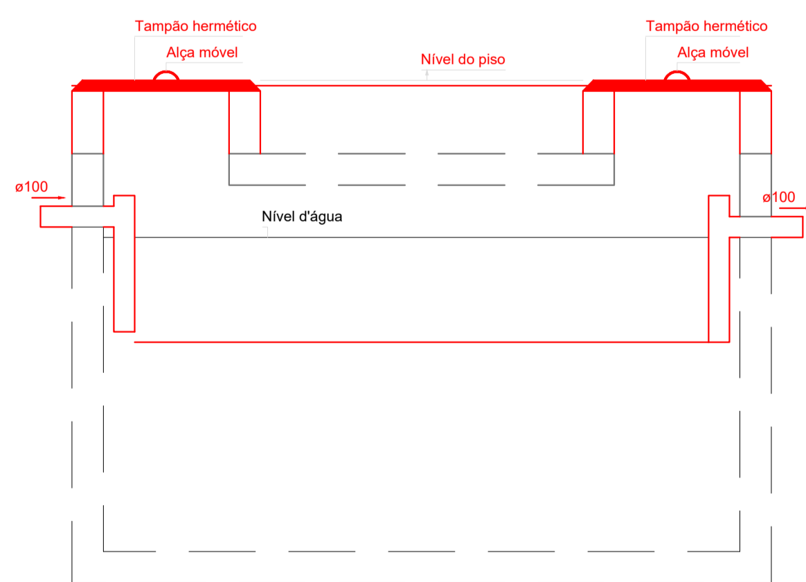
CORTE - TANQUE SÉPTICO ESCALA: 1/25
