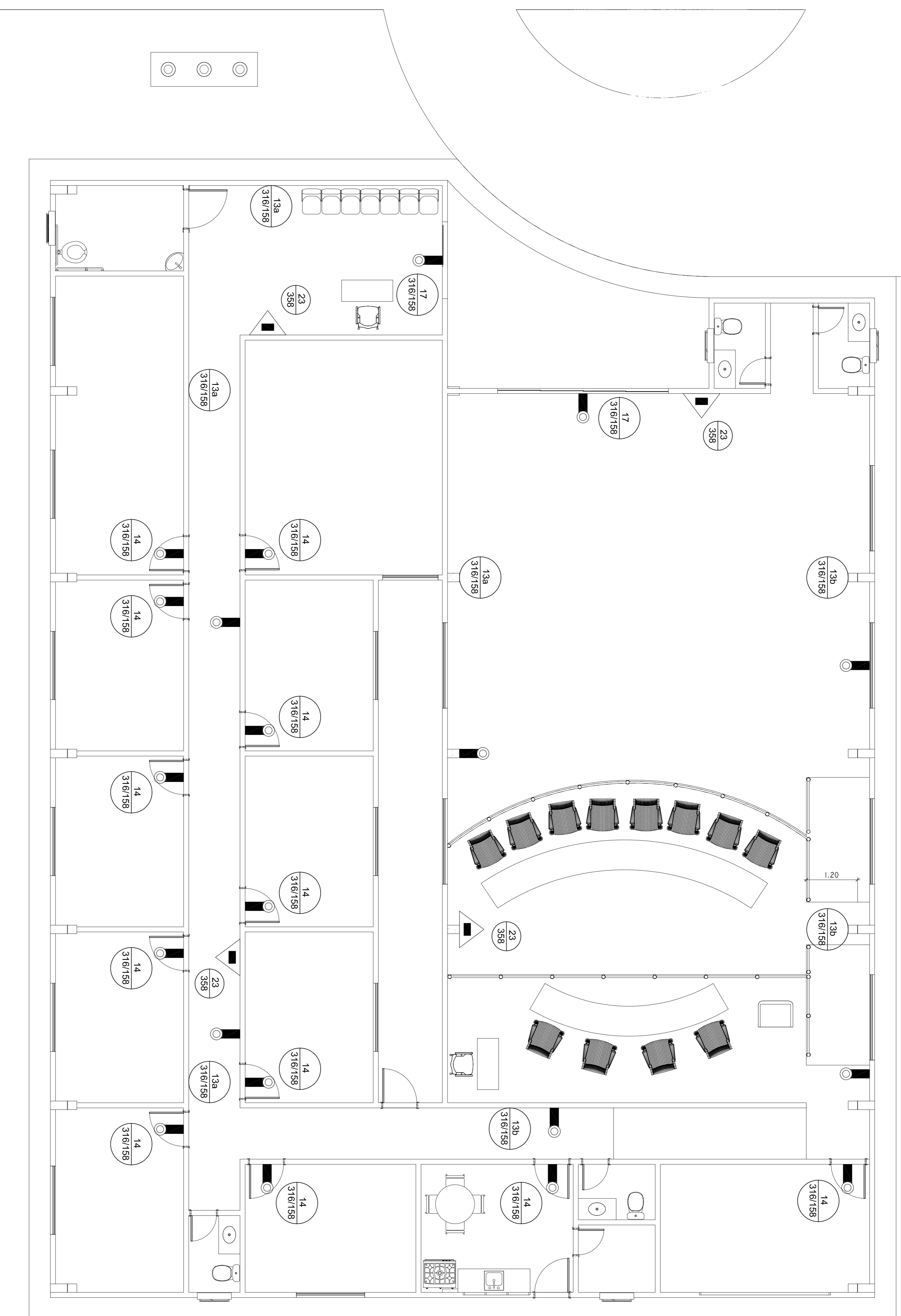
DETs. 01 e 02 - EXTINTOR E L. DE EMERGENCIA S/ESC.
