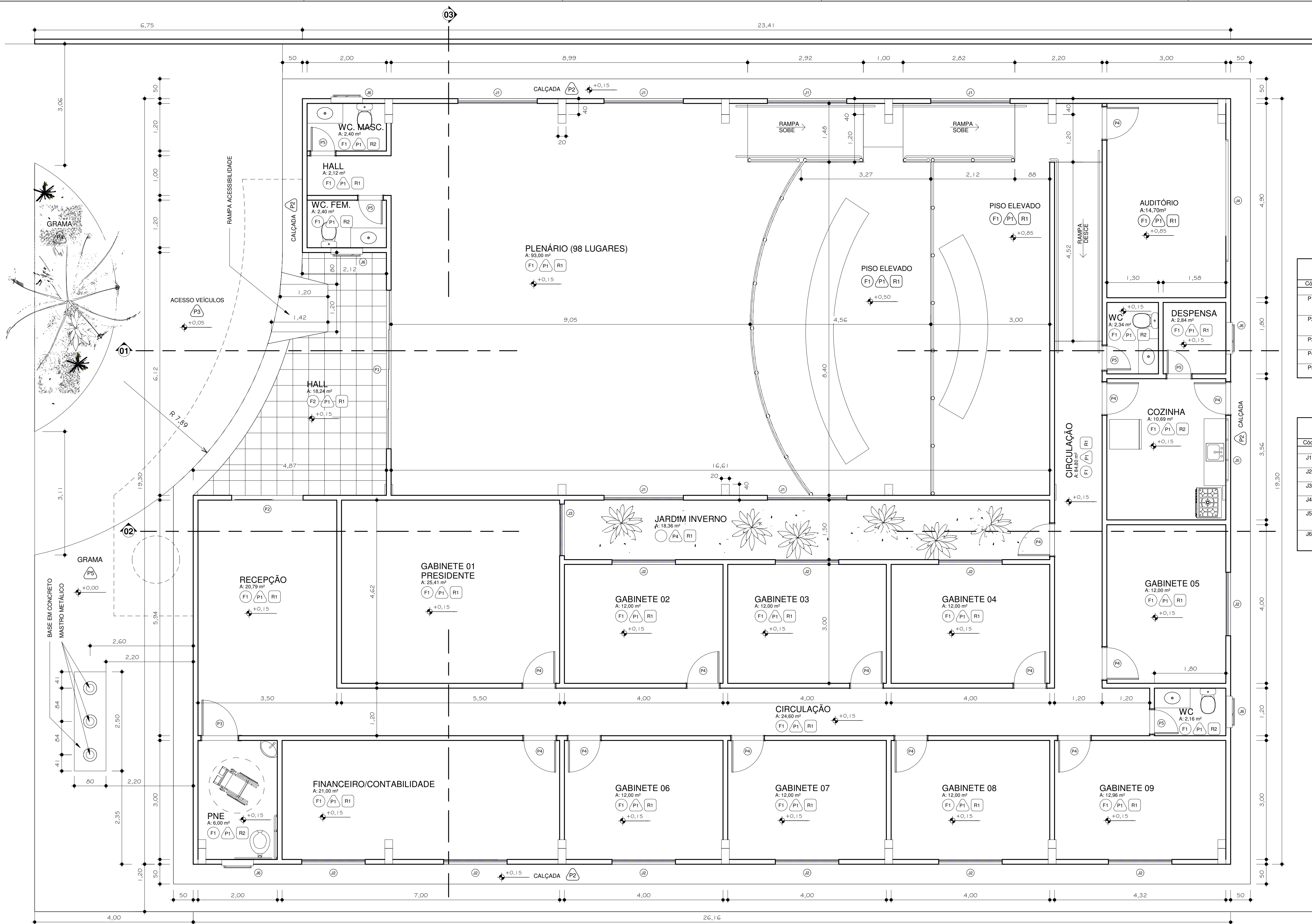
1 PLANTA BAIXA 1 : 50
